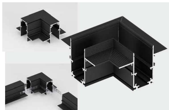
MC01-3 УГОЛ КОРПУСА МАГНИТНОГО ШИНОПРОВОДА ДЛЯ ГКЛ (13,5 ММ)
