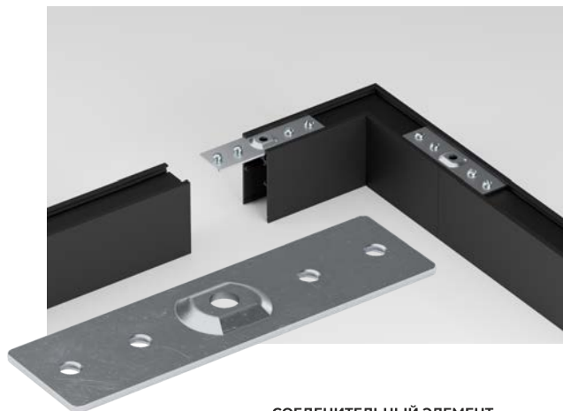
MP01-1 СОЕДИНИТЕЛЬНЫЙ ЭЛЕМЕНТ КОРПУСА МАГНИТНОГО ШИНОПРОВОДА «F»
